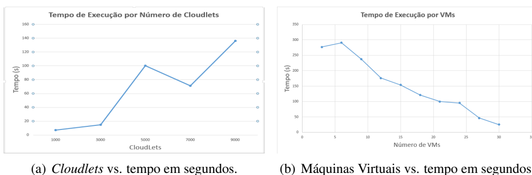
Figura 5. Sistema Localizador de Etiquetas no CloudSim .
