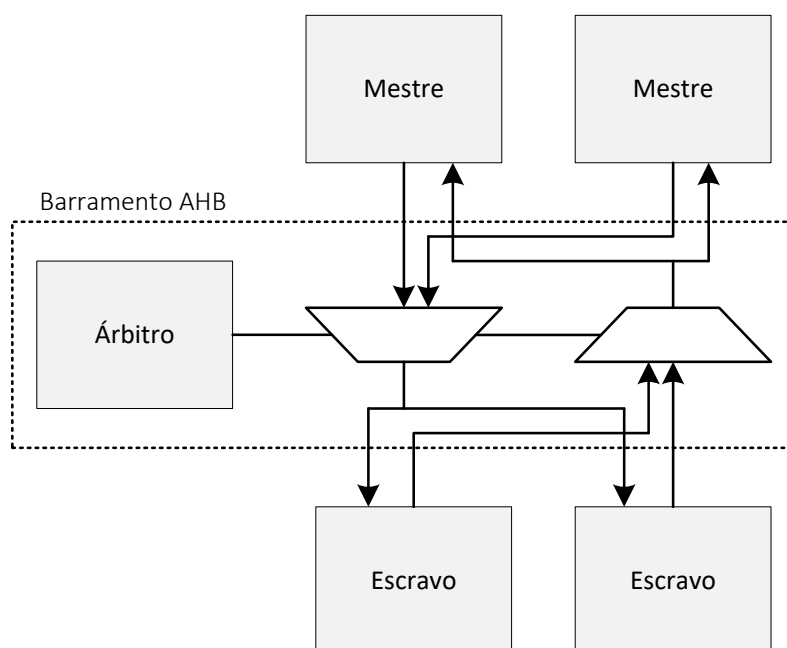
Figura 1. Interconexão do barramento AHB
