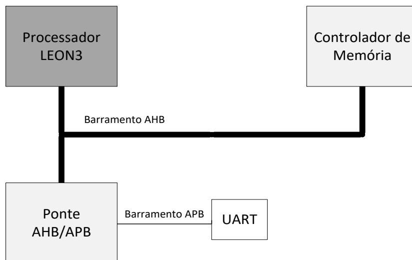
Figura 4. Arquitetura de sistema padrão
