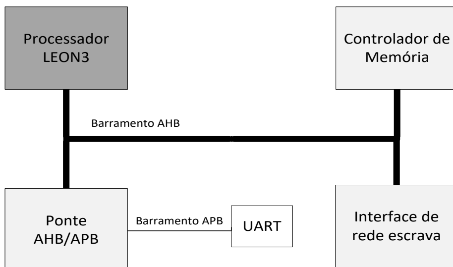
Figura 7. Arquitetura com interface de rede conectada ao barramento
