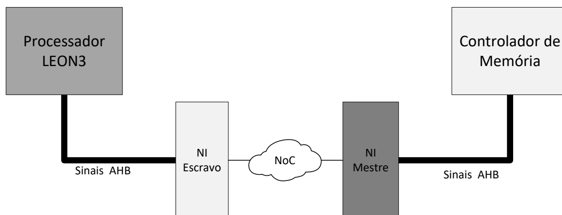
Figura 8. Arquitetura com interface de rede conectada ao processador
