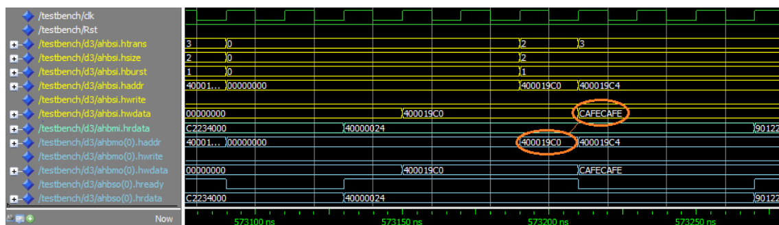
Figura 5. Simulação de transferência simples
