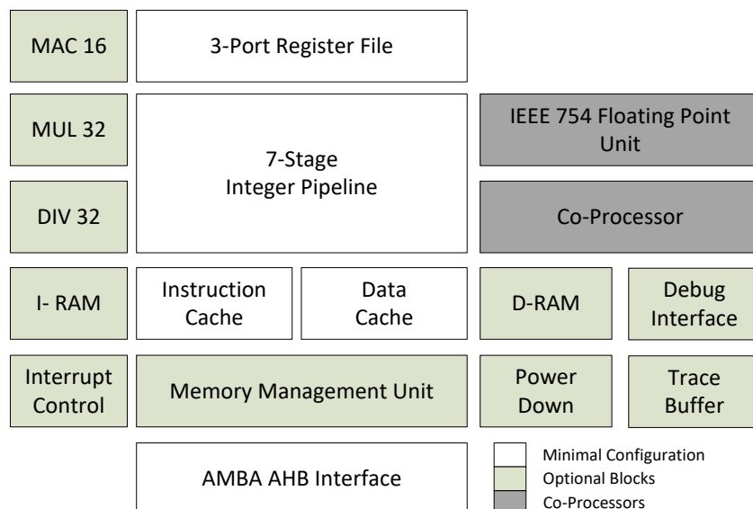
Figura 2. Diagrama de blocos do LEON3
