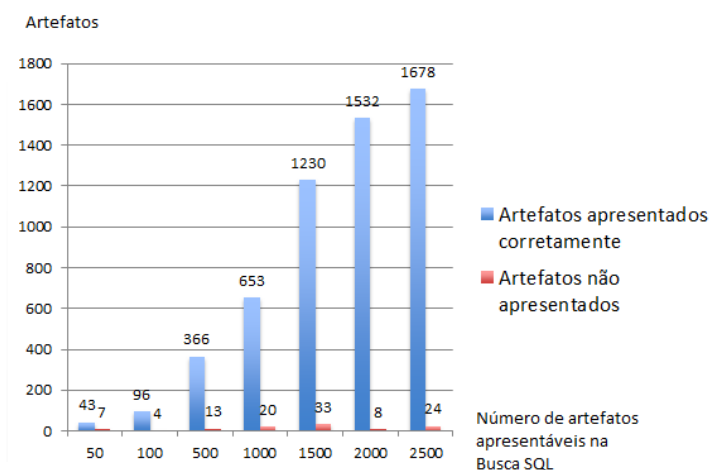
Figura 5 – Número de artefatos apresentados e não apresentados pelos mecanismos de busca SQL e com algoritmo genético.
