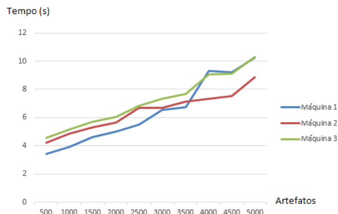
Figura 6 – Tempo de processamento em decorrência da quantidade avaliada de artefatos.
