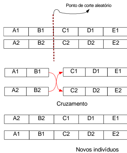
Figura 3 – Representação esquemática de cruzamento de indivíduos
