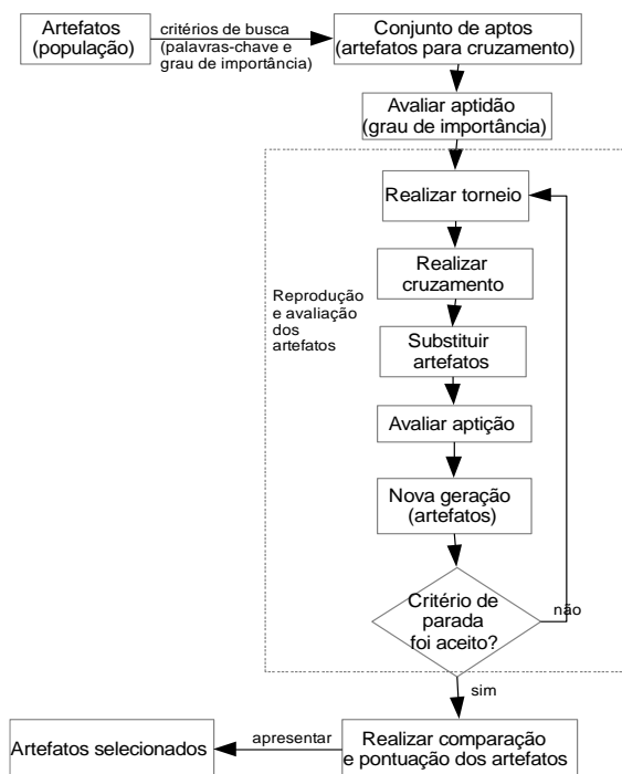
Figura 1 – Representação esquemática do algoritmo
