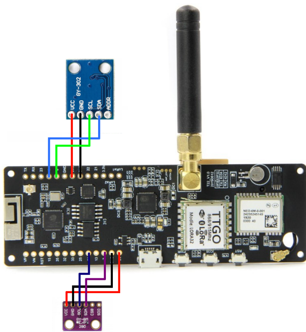
Figura 3: Integração dos sensores e módulos na solução baseada em ESP32 e LoRa
