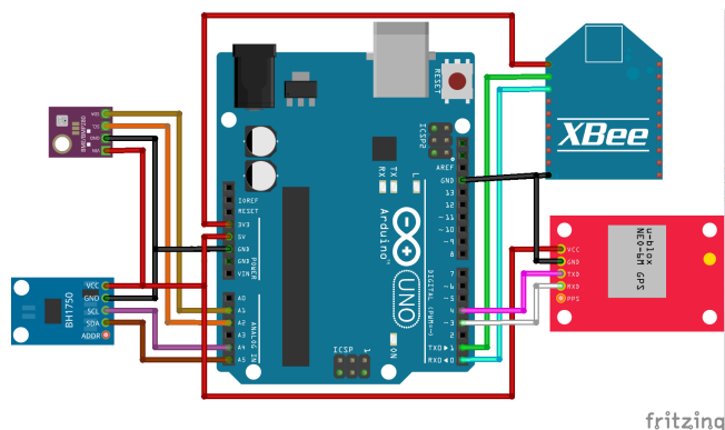
Figura 2: Integração dos sensores e módulos na solução baseada em Arduino e XBee
