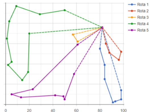
Figura 1: Ilustração de um PRV com 5 veículos e 31 clientes.
