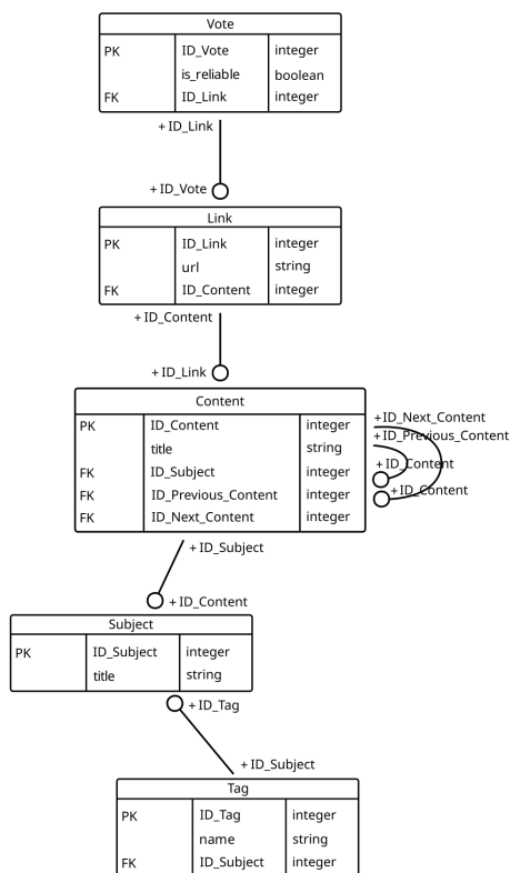
Figura 2: Diagrama de entidade-relacionamento do banco de dados.
