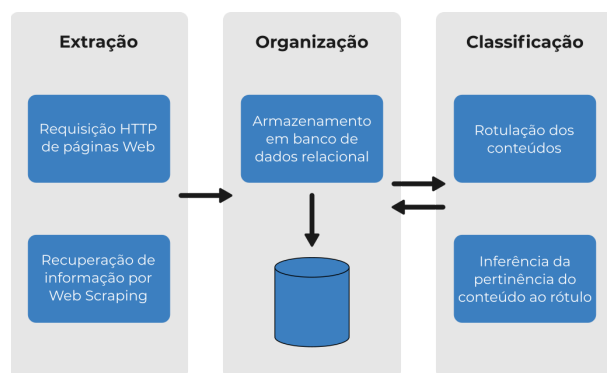
Figura 1: Diagrama de representação das responsabilidades dos módulos.
