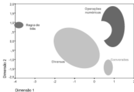
Figura 1: Diagrama produzido pela análise MDS do pacote estatístico SPSS, mostrando o agrupamento dos sujeitos em função da semelhança de estratégias utilizadas na resolução dos problemas.
